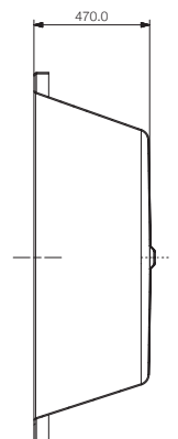
Section A-A
